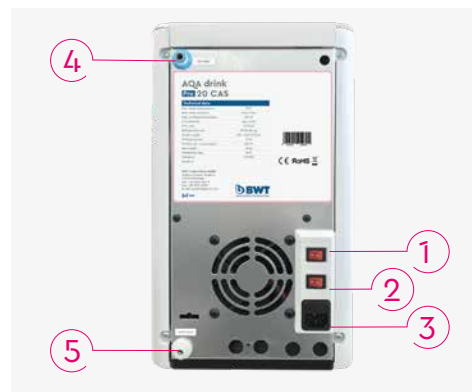
Afb. 3: Paneel aan de achterkant van de AQA drink Pro 20 CAS
