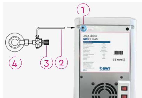
Afb. 8: De CO 2 gascilinder aansluiten
