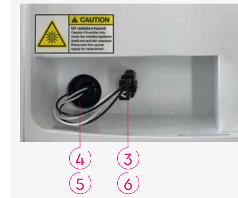
Abb. 9: Öffnung der UV-Lampe unter dem Deckel von AQA drink Pro 20
